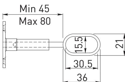
REGGITUBO OVALE REGOLABILE IN ZAMA
