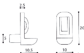
REGGICRISTALLO A POLTRONCINA A SCATTO
