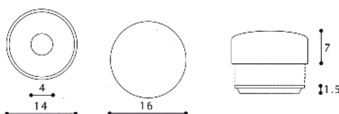
COPRIVITE A SCATTO IN PLASTICA
