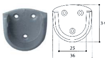
REGGITUBO 25MM IN PLASTICA
