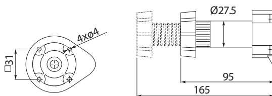
PIEDE PER CUCINA REGOLABILE
