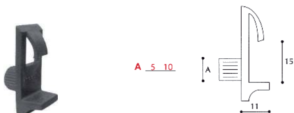
REGGIMENSOLA A POLTRONCINA A SCATTO
