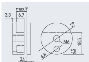
MENSOLINA REGGISPECCHIO IN ZAMA
