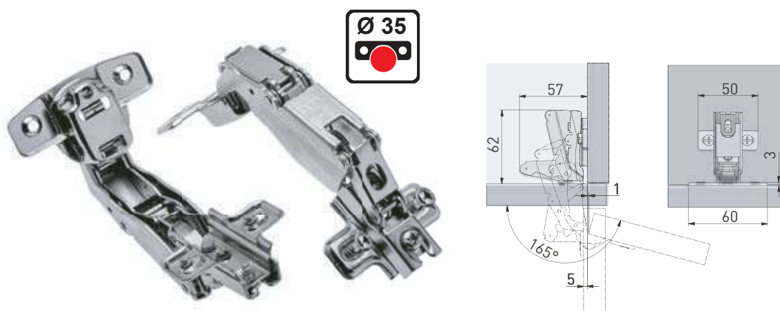
CERNIERA A SCATTO IN ACCIAIO A 165°
