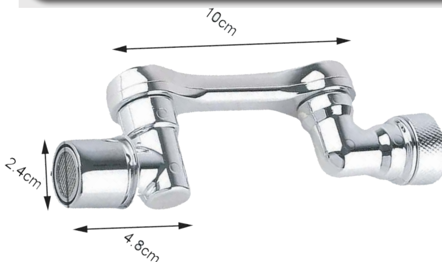
RUBINETTO RUOTABILE A 1080° IN METALLO CROMATO
