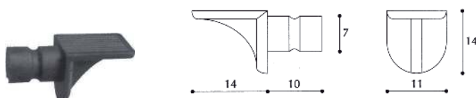
REGGIMENSOLA SPOSTABILE
