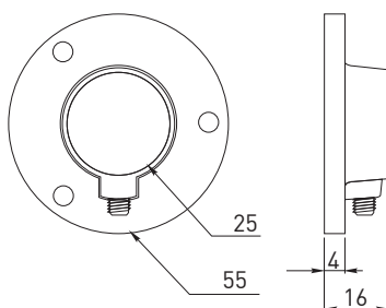
SUPPORTO TONDO IN ACCIAIO PER TUBO
