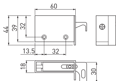
ATTACCAGLIA PER PENSILI (90KG)
