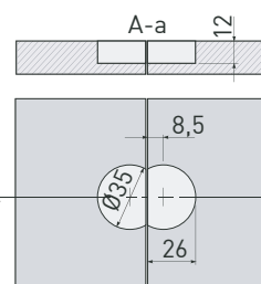
CERNIERA PER RIBALTA
