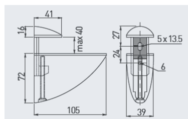
REGGIMENSOLA "PELIKAN GRANDE" IN ZAMA
