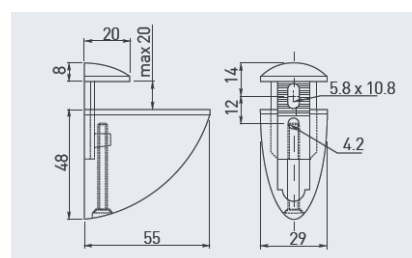
REGGIMENSOLA "PELIKAN PICCOLO" IN ZAMA
