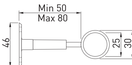
REGGITUBO TONDO APERTO REGOLABILE IN ZAMA
