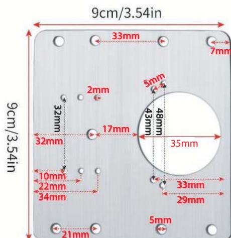
PIASTRA IN ACCIAIO DI RIPARAZIONE PER PENSILI
