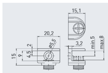
REGGICRISTALLO "BABY" IN ZAMA
