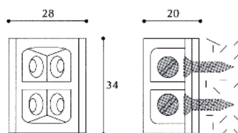
GIUNZIONE ANGOLARE IN PLASTICA
