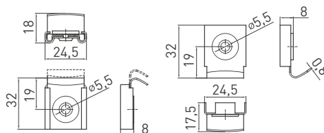
SUPPORTI REGGISPECCHIO CON MOLLA
