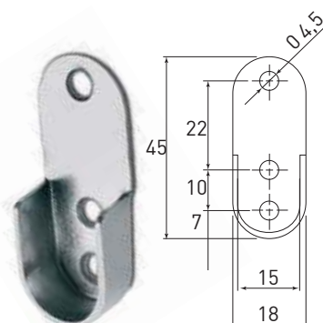
REGGITUBO RDR IN ACCIAIO PER TUBI DA Ø15
